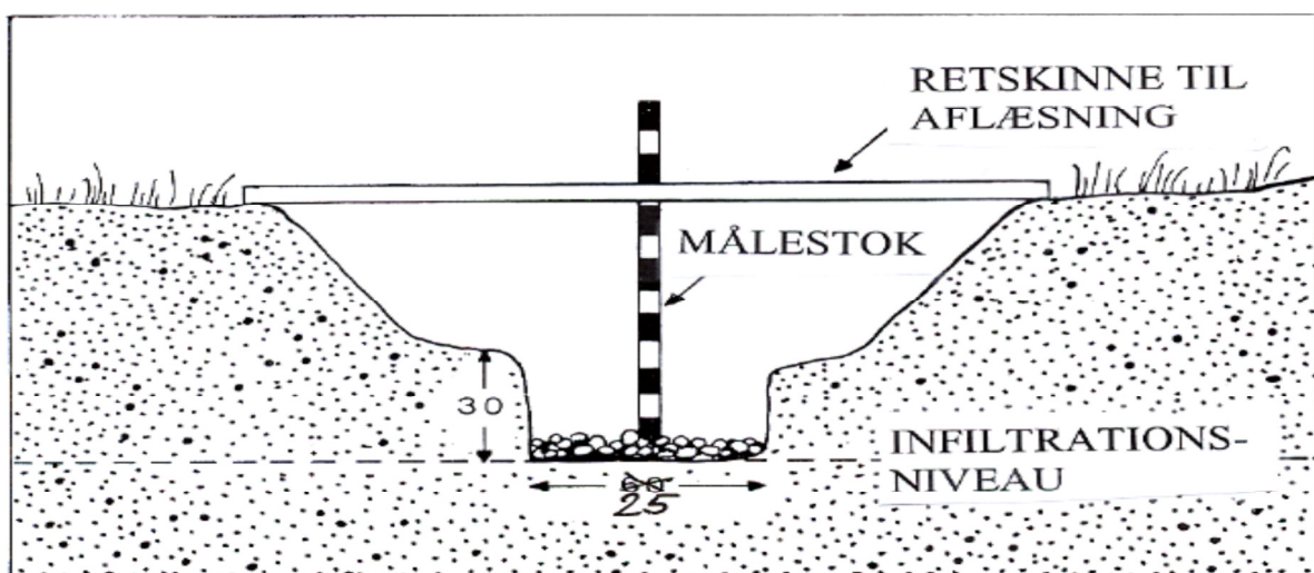
Figur 1. Skitse af prøvehul til udførelse af nedsivningstest /2/.
