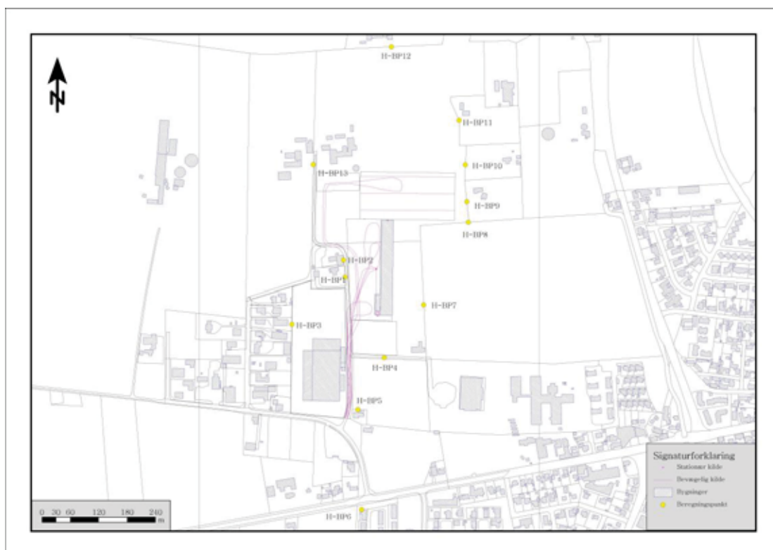
Figur 3: Placering af beregningspunkter omkring den planlagte huldækfabrik.
