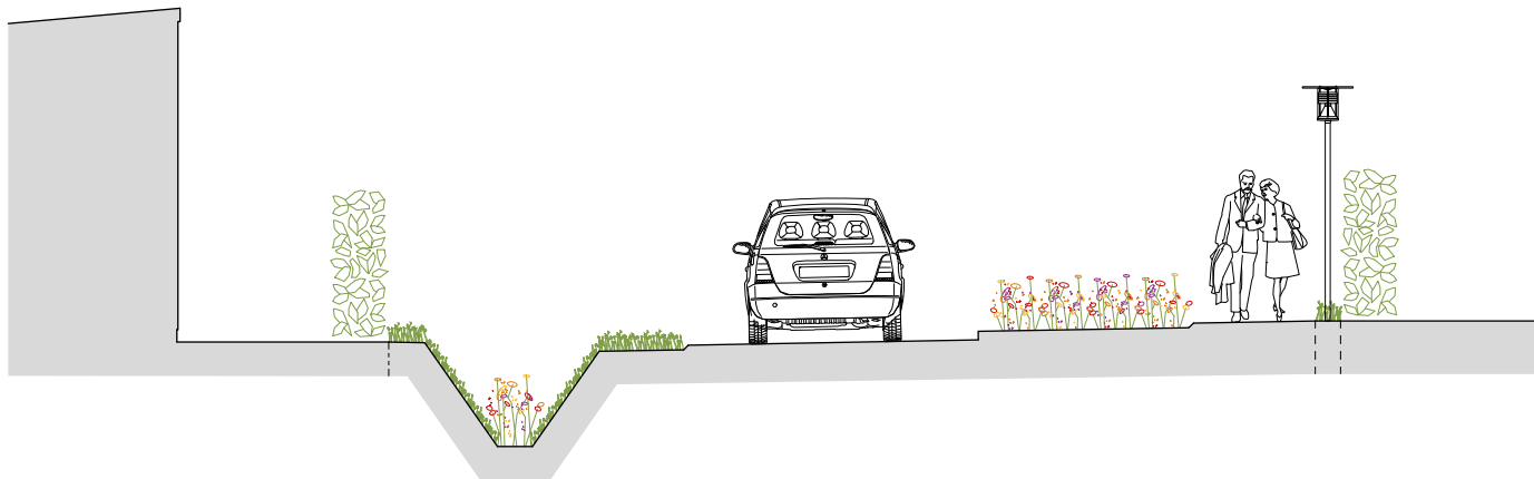
SNIT A-a - 1:100 FORDELINGSVEJ KÆRBLOMST ALLÉ
